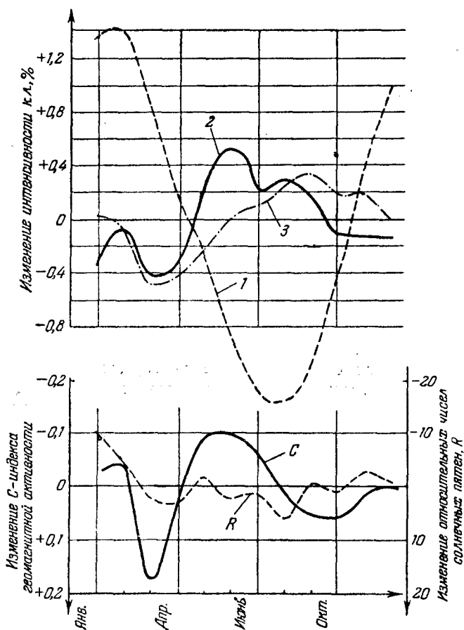
Рис. 9. Годовые вариации космических лучей и магнитная активность. 1 — измерения (Челтенхэм); 2 — метеорологический эффект исключён (Челтенхэм); 3 — измерения (Гуанкайю); C — индекс магнитной активности (левая шкала); R — относительные числа солнечных пятен, числа Вольфа (правая шкала).
